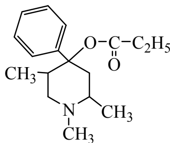
промедол
