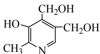
пиридоксол
