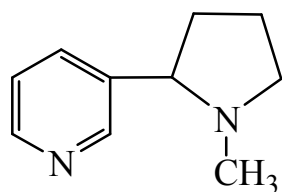
никотин
