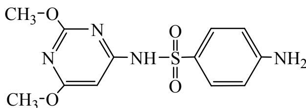
сульфадиметоксин
