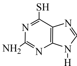
тиогуанин
