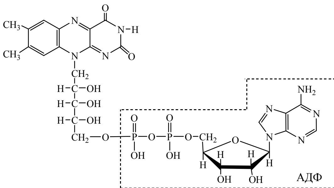
флавинадениндинуклеотид (ФАД)
