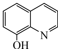
оксин
