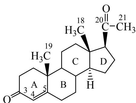
прогестерон
