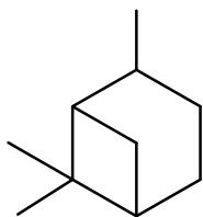
пинан
