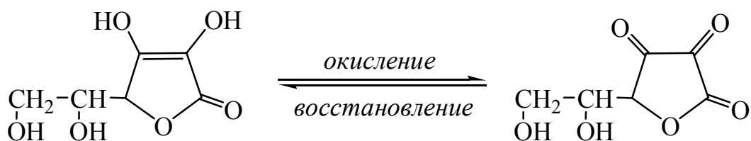
аскорбиновая кислота
