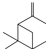
\beta -пинен
