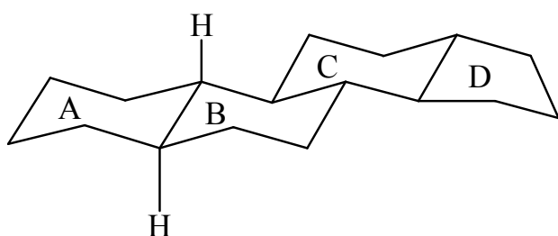
транс-гонан
