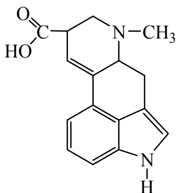
лизергиновая кислота
