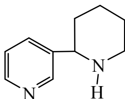
анабазин
