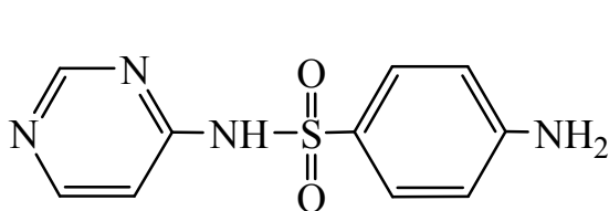
сульфазин
