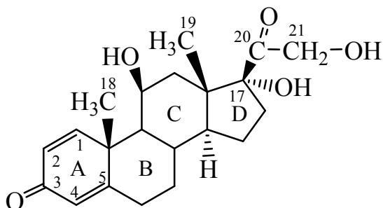
преднизолон
