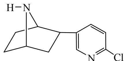
эпибатидин
