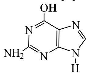
гуанин
