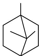
борнан
