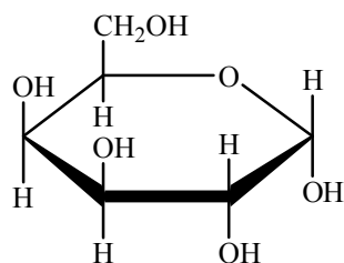
\alpha -D-галактопираноза
