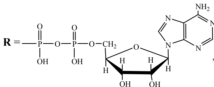
флавинадениндинуклеотид (ФАД).
