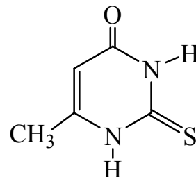
метилтиоурацил
