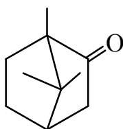
камфора
