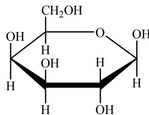
\beta -D-галактопираноза
