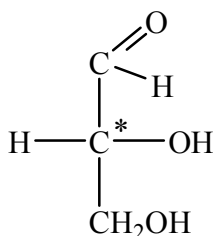
D-глицериновый альдегид
