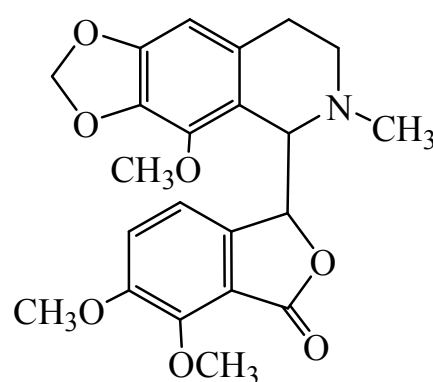
наркотин
