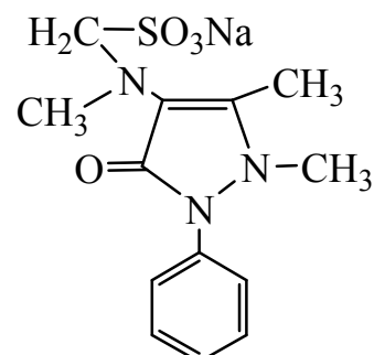
анальгин
