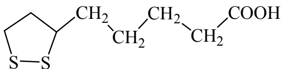
липоевая кислота
