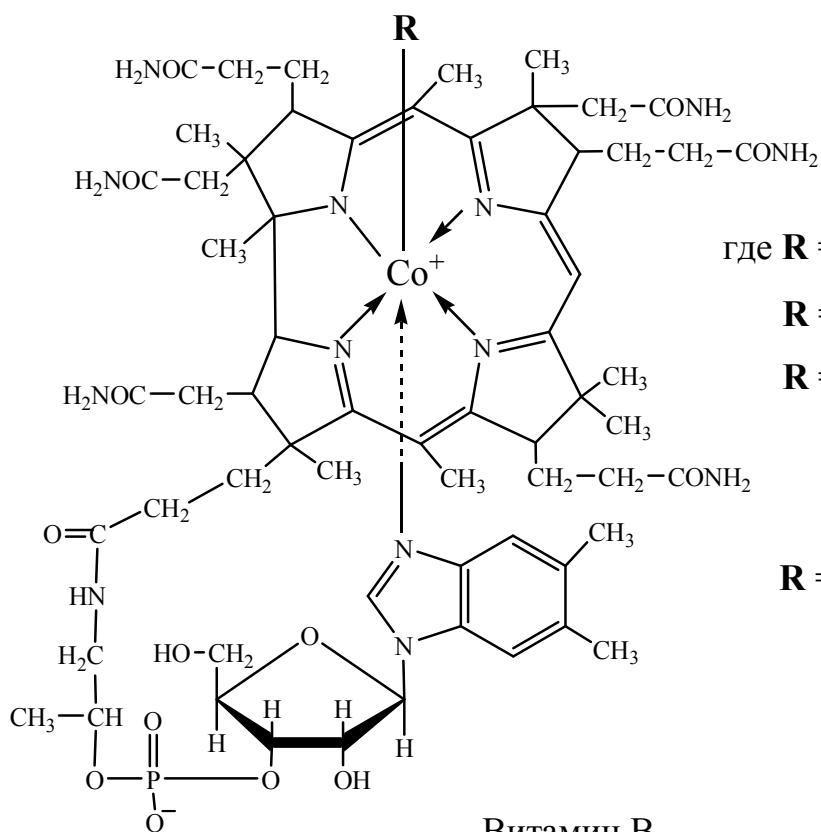
Витамин В 12
