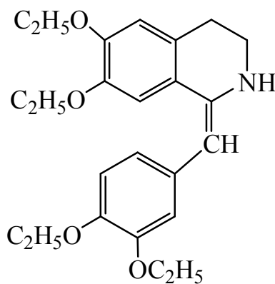
но-шпа
