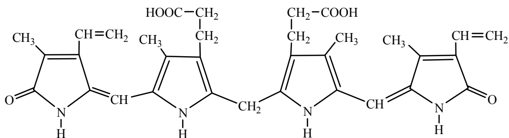
билирубин
