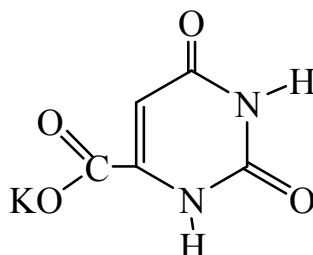
оротат калия
