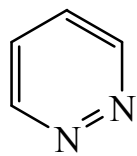
пиридазин
