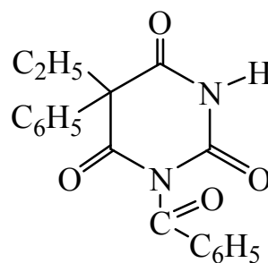
бензонал
