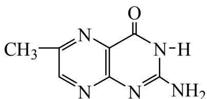
2-амино-6-метил- -4-оксоптеридин
