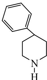
4-фенилпиперидин
