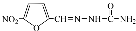
фурацилин
