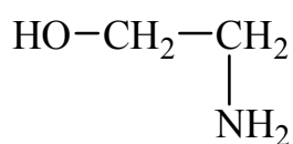
коламин
