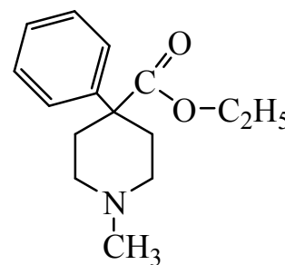
лидол
