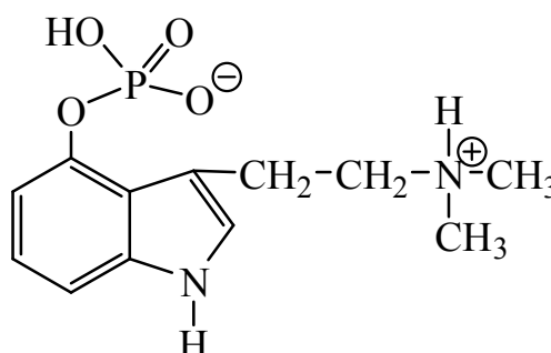
псилоцибин
