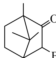
бромкамфора
