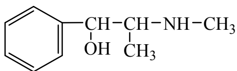
эфедрин
