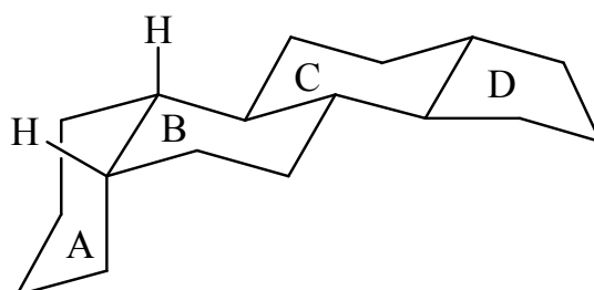
цис-гонан
