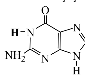
гуанин
