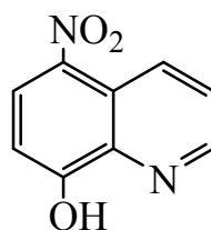
5-НОК
