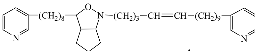
пиринодемин А
