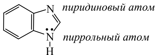
бензимидазол
