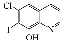
энтеросептол
