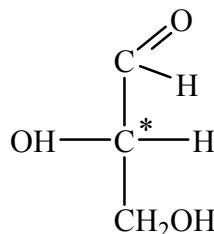
L-глицериновый альдегид
