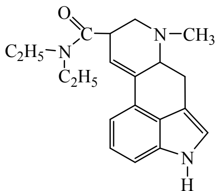
ЛСД
