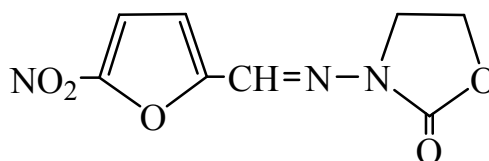
фуразолидон
