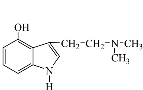
псилоцин
