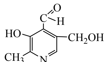
пиридоксаль
