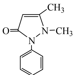
антипирин
