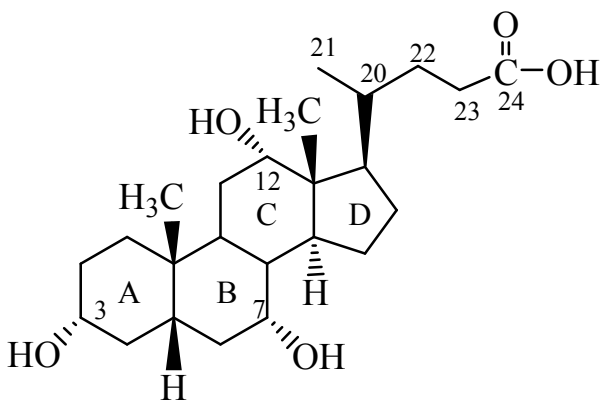
холевая кислота
