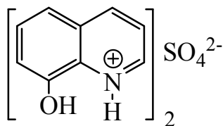
хинозол
