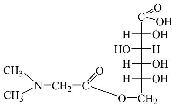
пангамовая кислота
