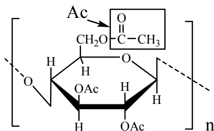
ацетат целлюлозы
