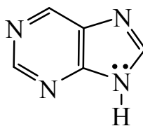
пурин
