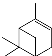
\alpha -пинен
