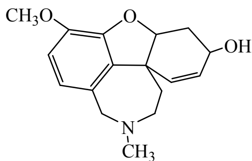
галантамин
