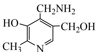
пиридоксамин
