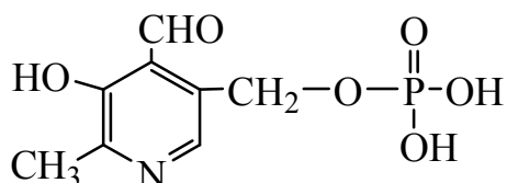
пиридоксальфосфат
