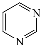
пиримидин
