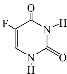
фторурацил
