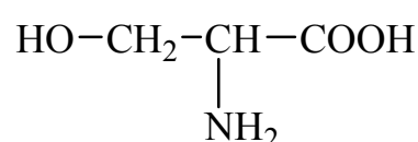
серин
