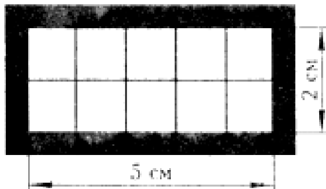
Рис. 2. Сеточка Раменского
